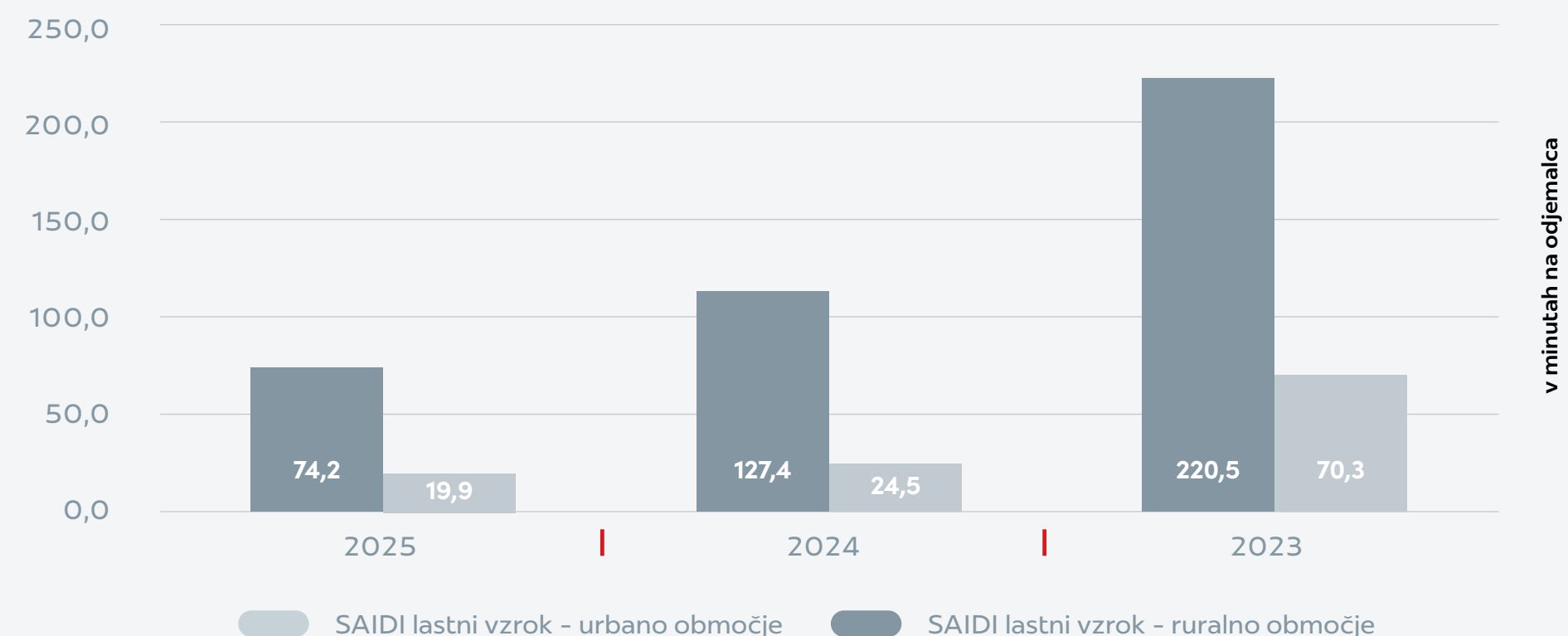
Graf 16: SAIDI zaradi lastnega vzroka, ločeno za urbano in ruralno območje – povprečni čas nenačrtovanih prekinitev, daljših od treh minut, ko ni bilo dobave električne energije (povprečno na odjemalca)
