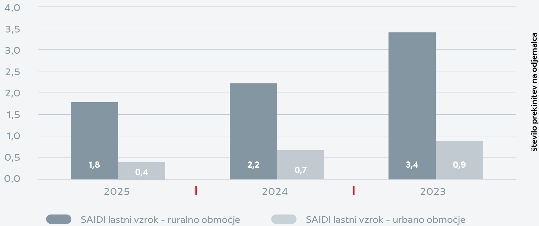
Graf 18: SAIFI zaradi lastnega vzroka, ločeno za urbano in ruralno območje – povprečno število nenačrtovanih prekinitev, daljših od treh minut (povprečno na odjemalca)
