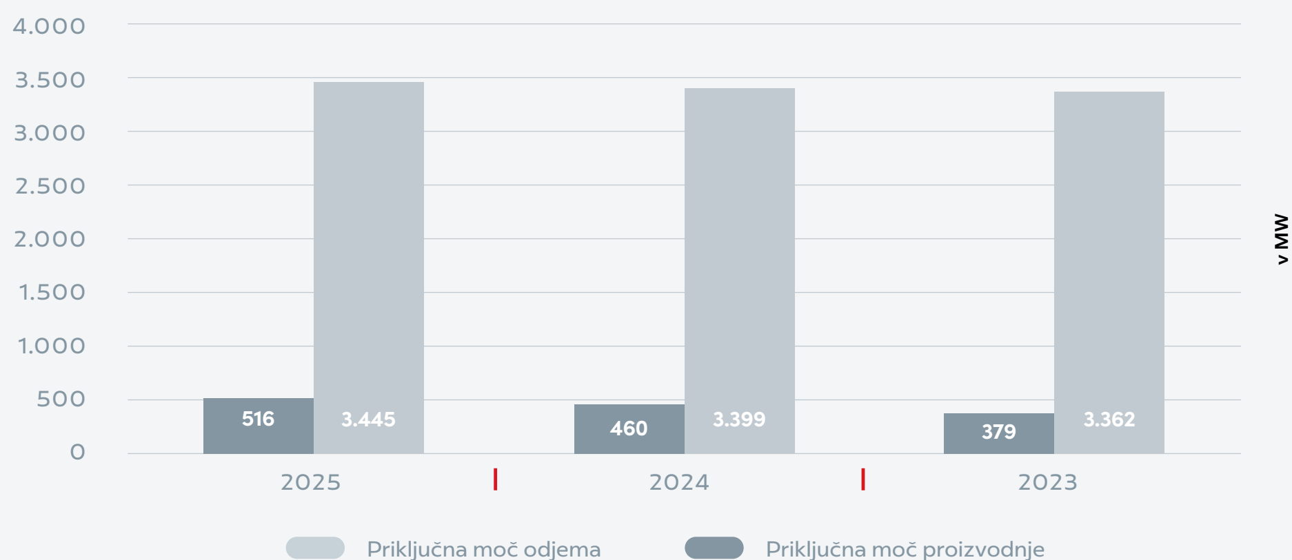
Graf 22: Priključna moč odjema in proizvodnje
